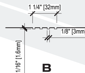
Détails : orifices de drainage
