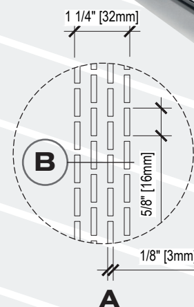
Détails : orifices de drainage
